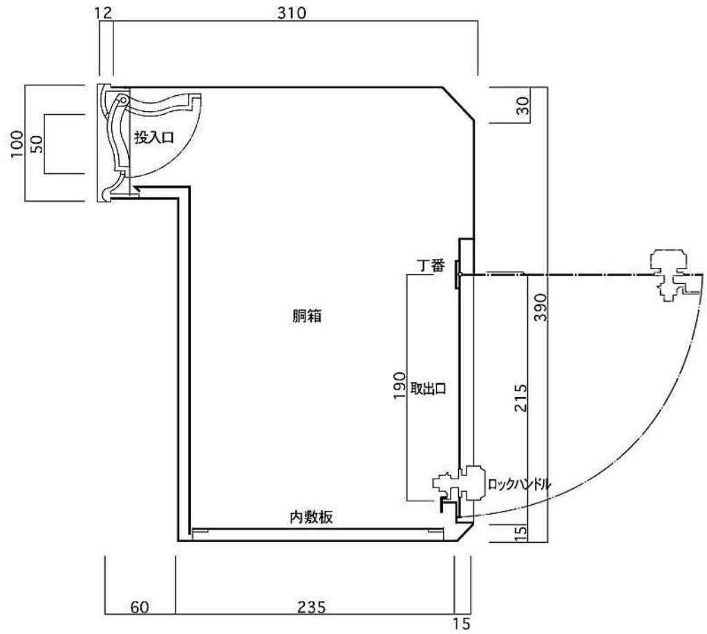
縦断面図
