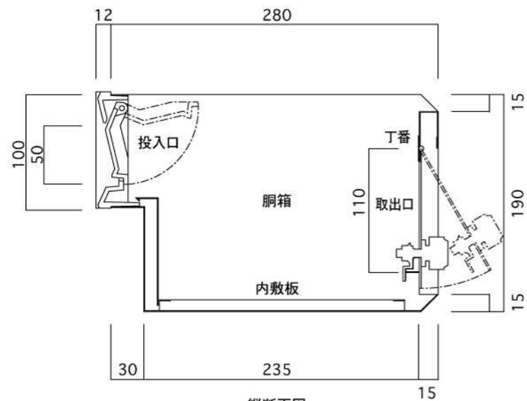
縦断面図
