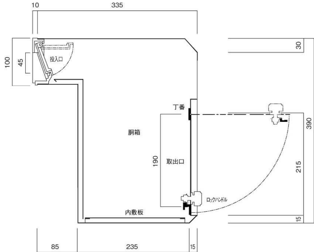
縦断面図
