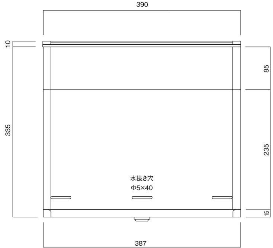
底面図
