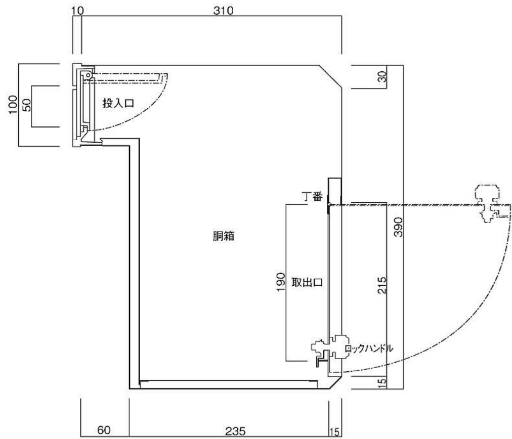
縦断面図
