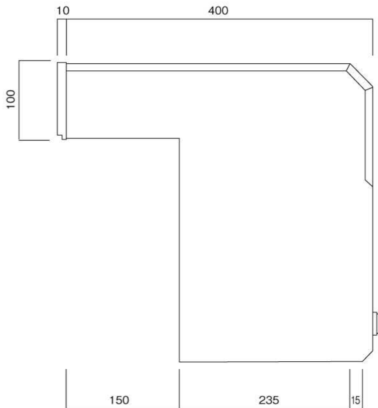
側面図
