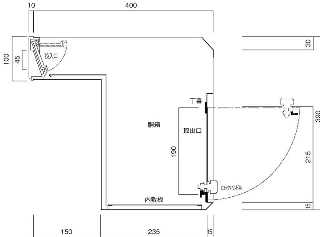
縦断面図
