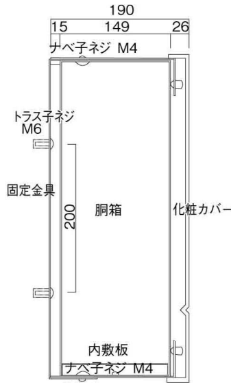
縦断面図
