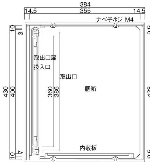
縦断面図
