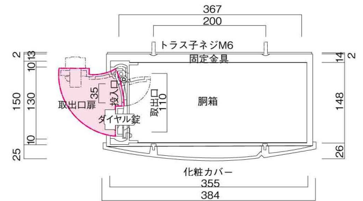
横断面図
