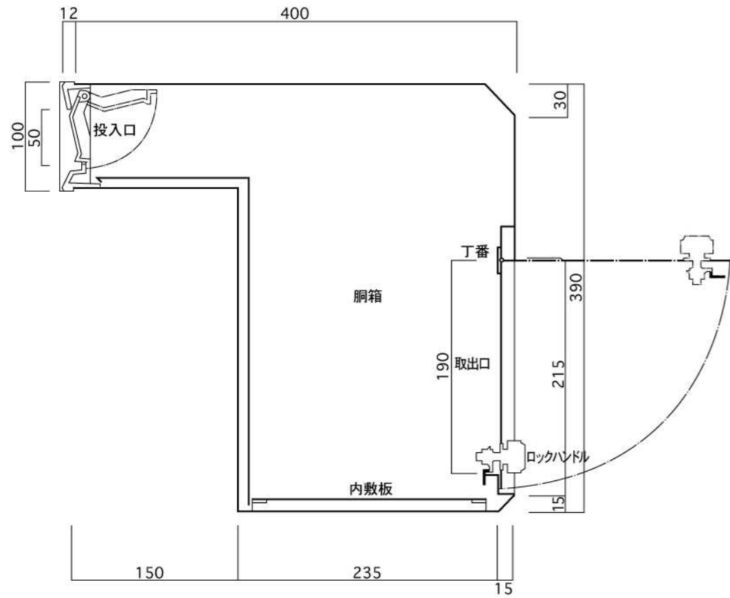
縦断面図
