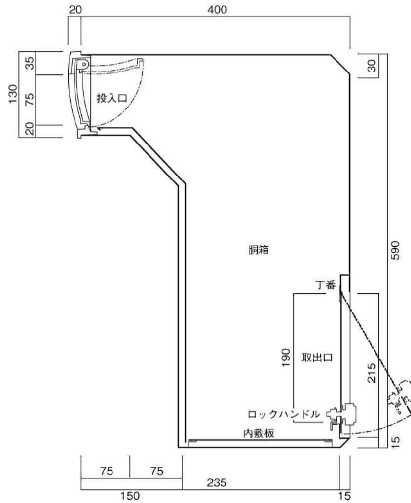
縦断面図
