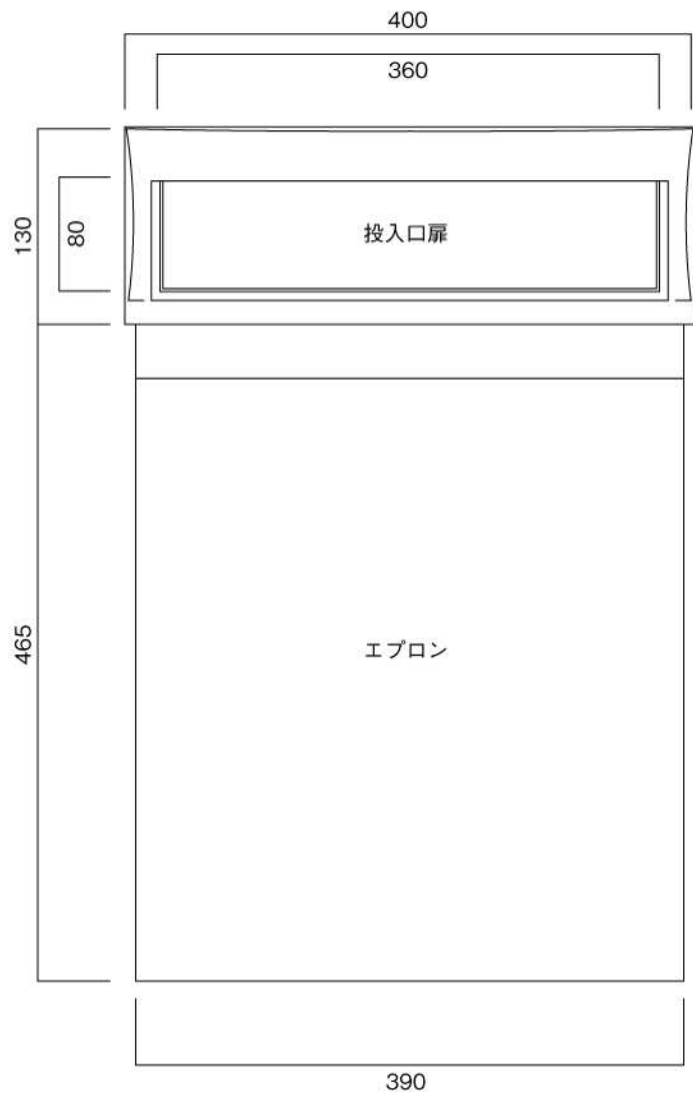
正面図
