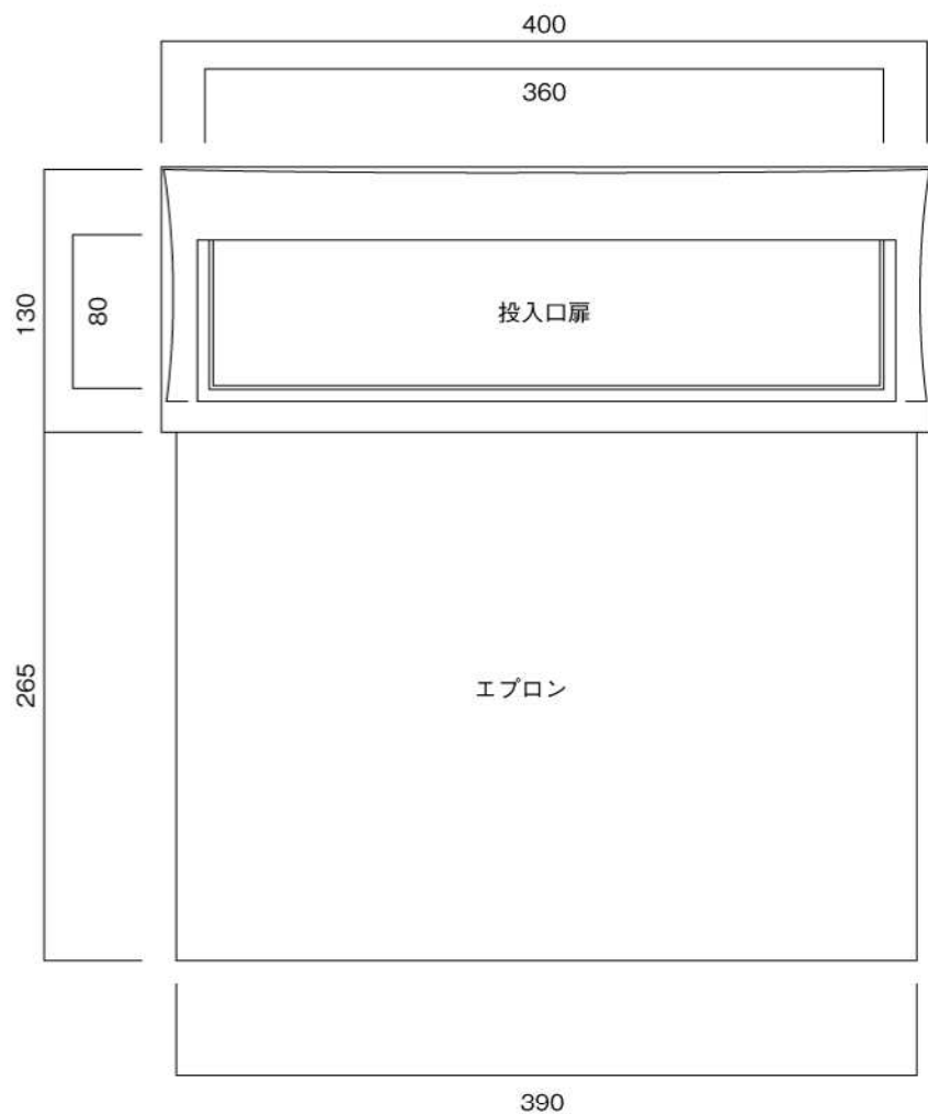
正面図
