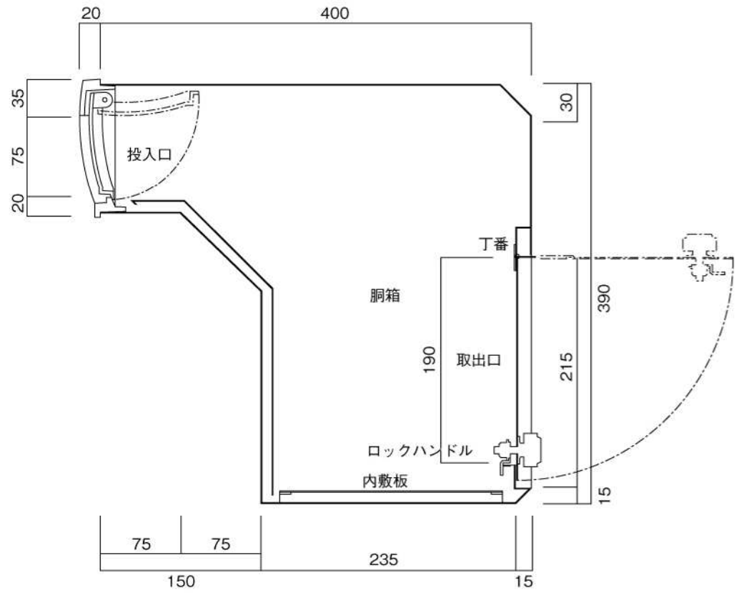
縦断面図
