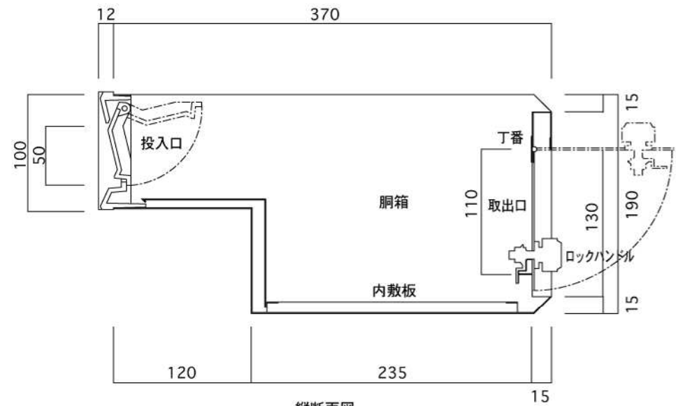
縦断面図
