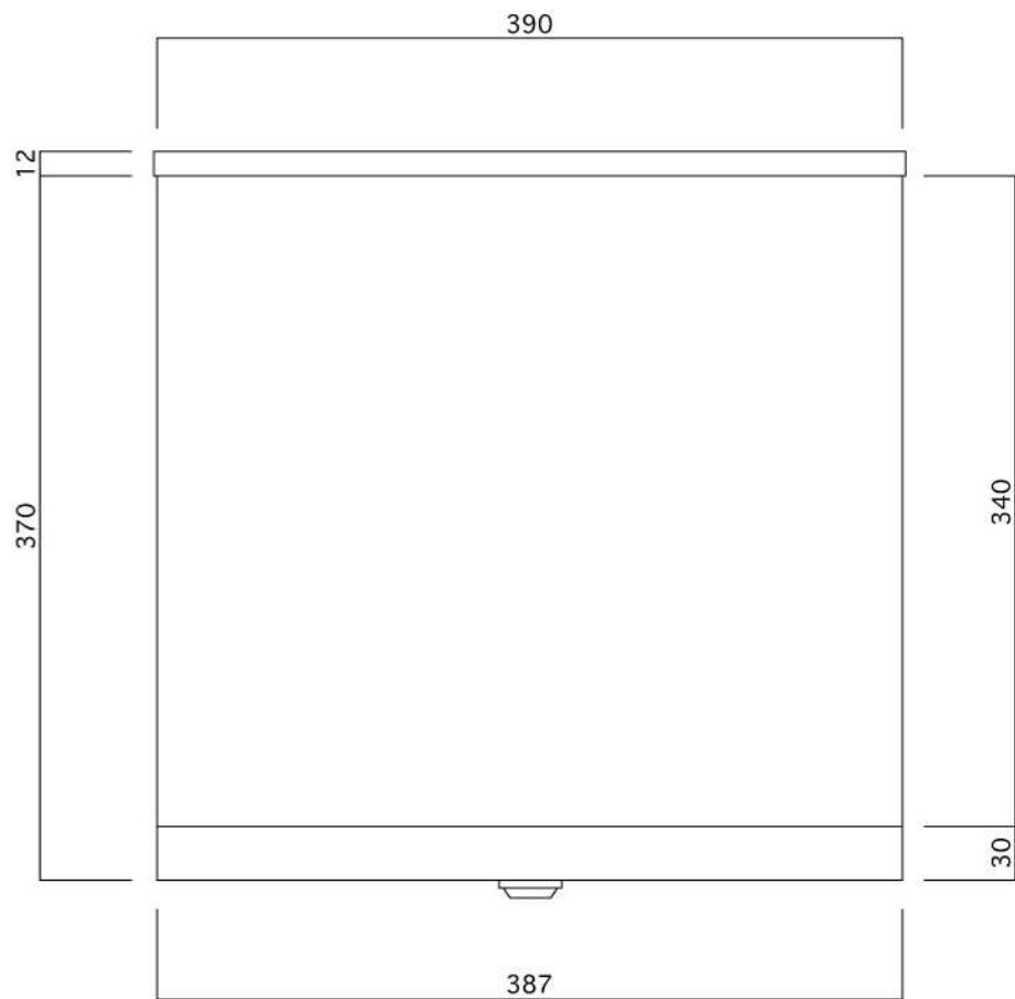
平面図
