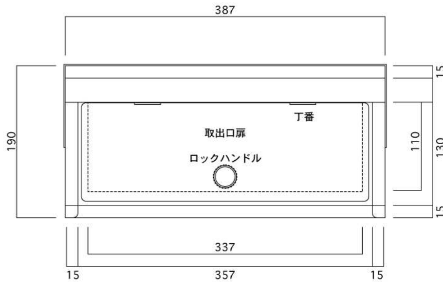
裏面図
