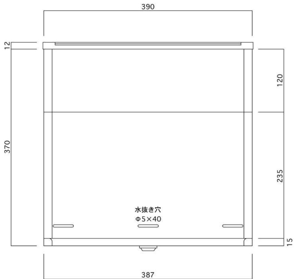
底面図
