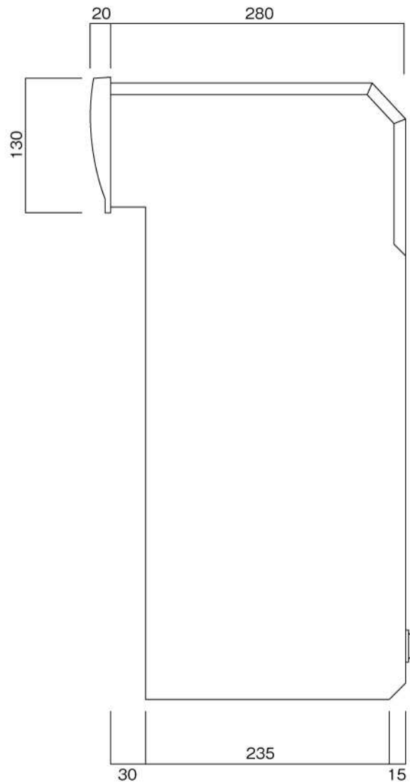
側面図
