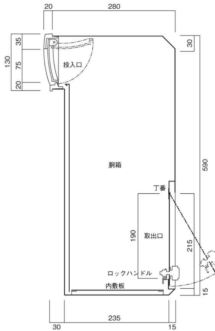
縦断面図
