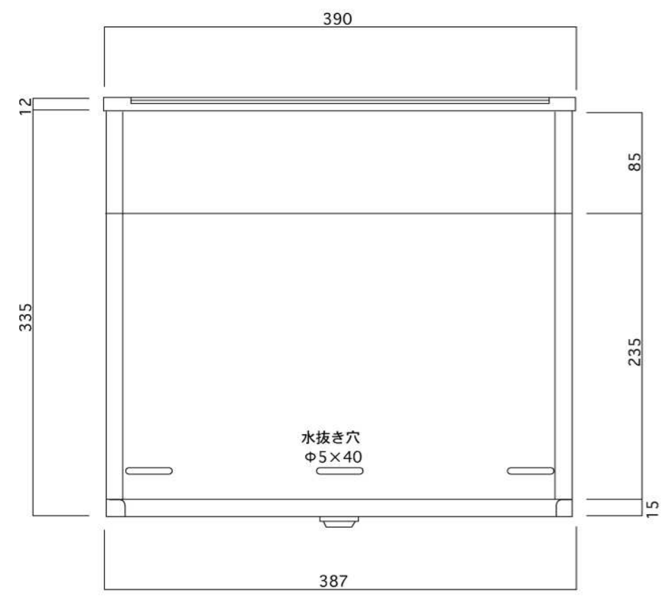
底面図
