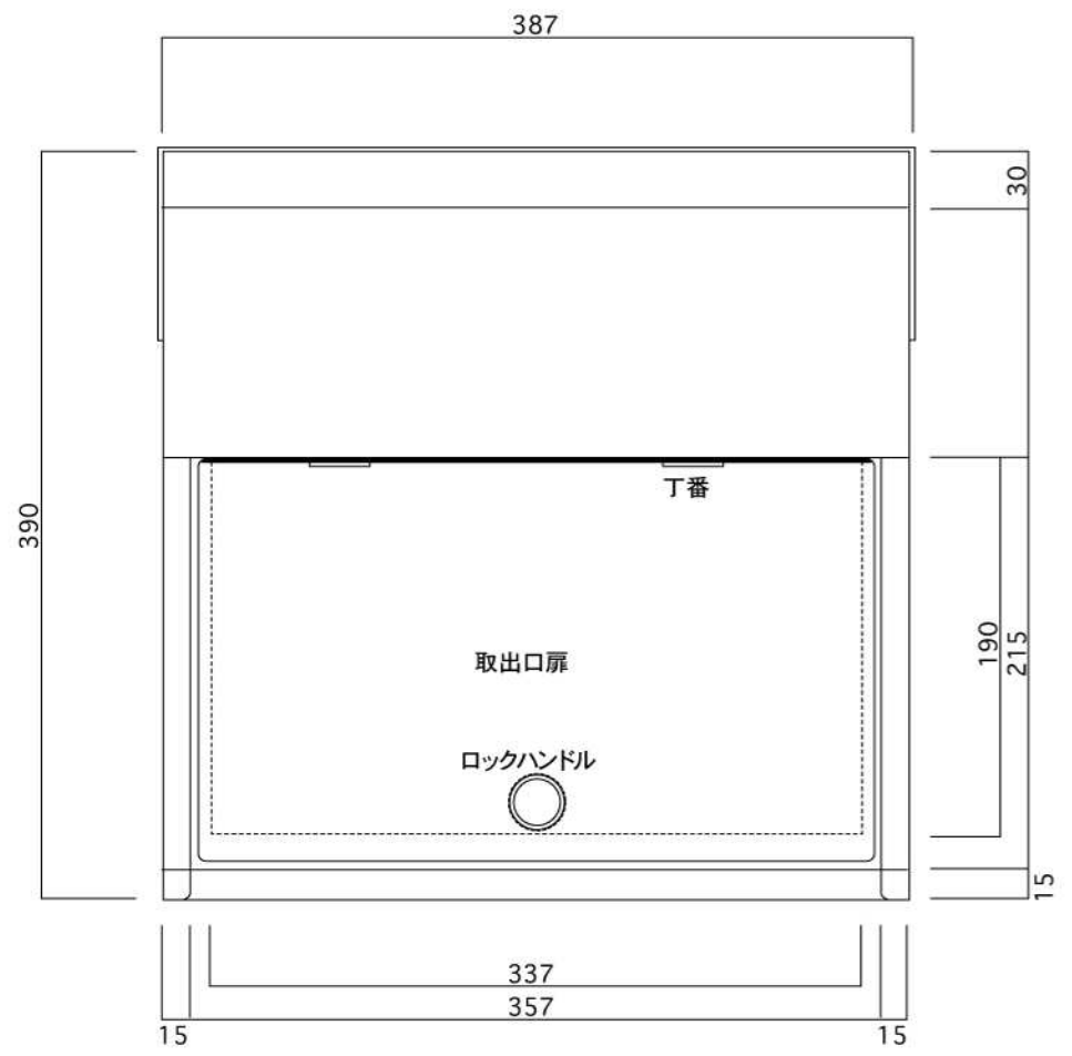
裏面図
