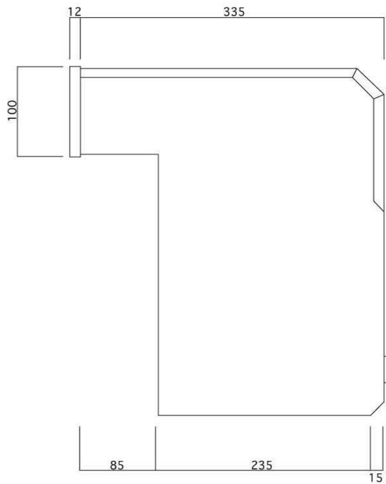
側面図
