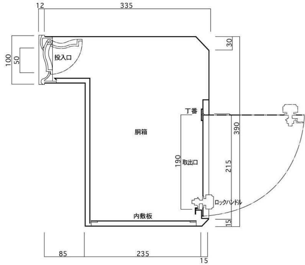
縦断面図
