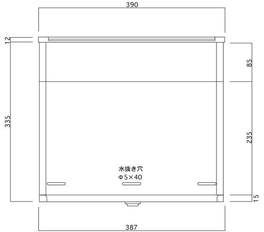
底面図
