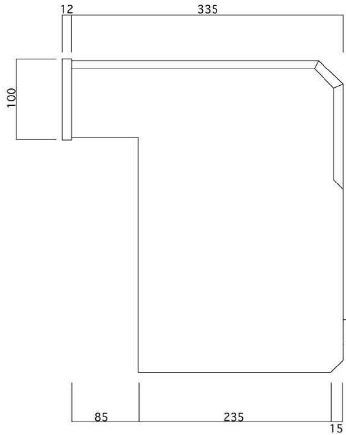
側面図
