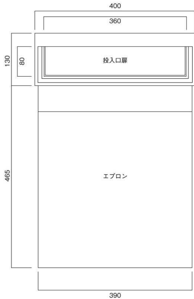
正面図
