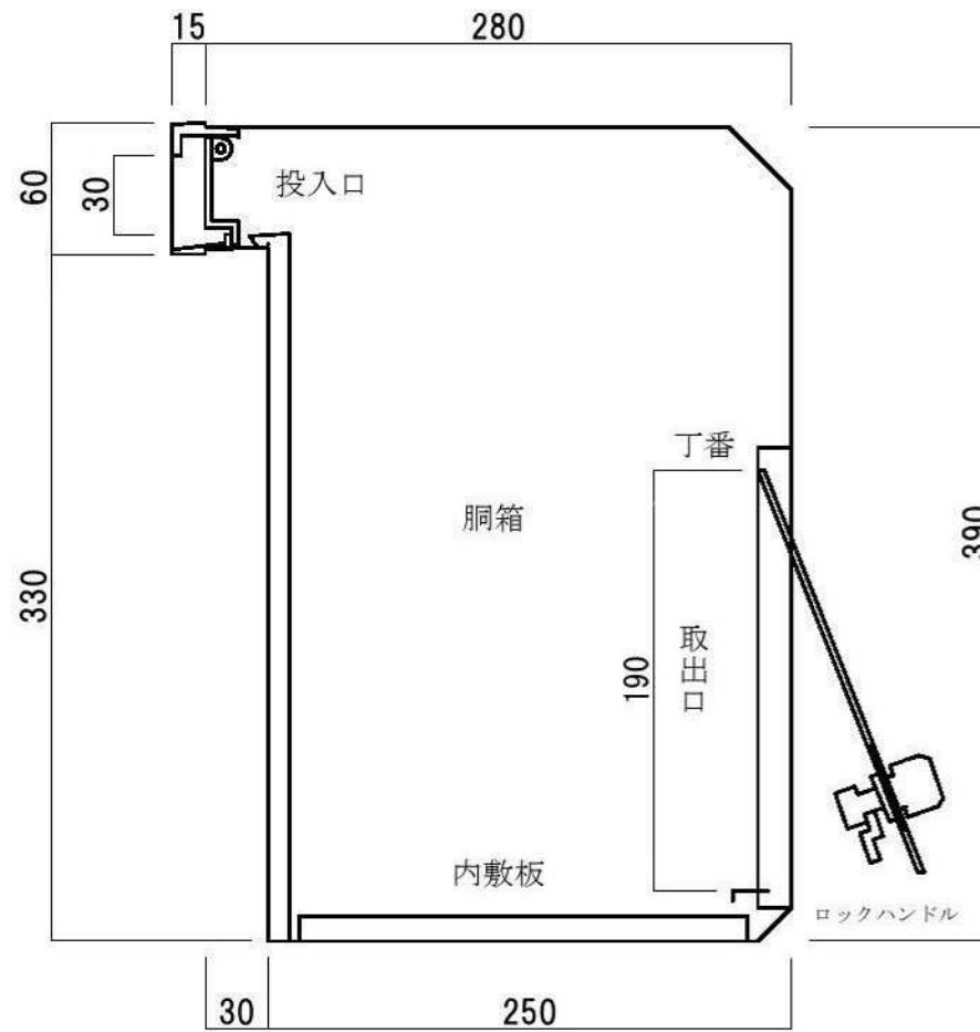
縦断面図
