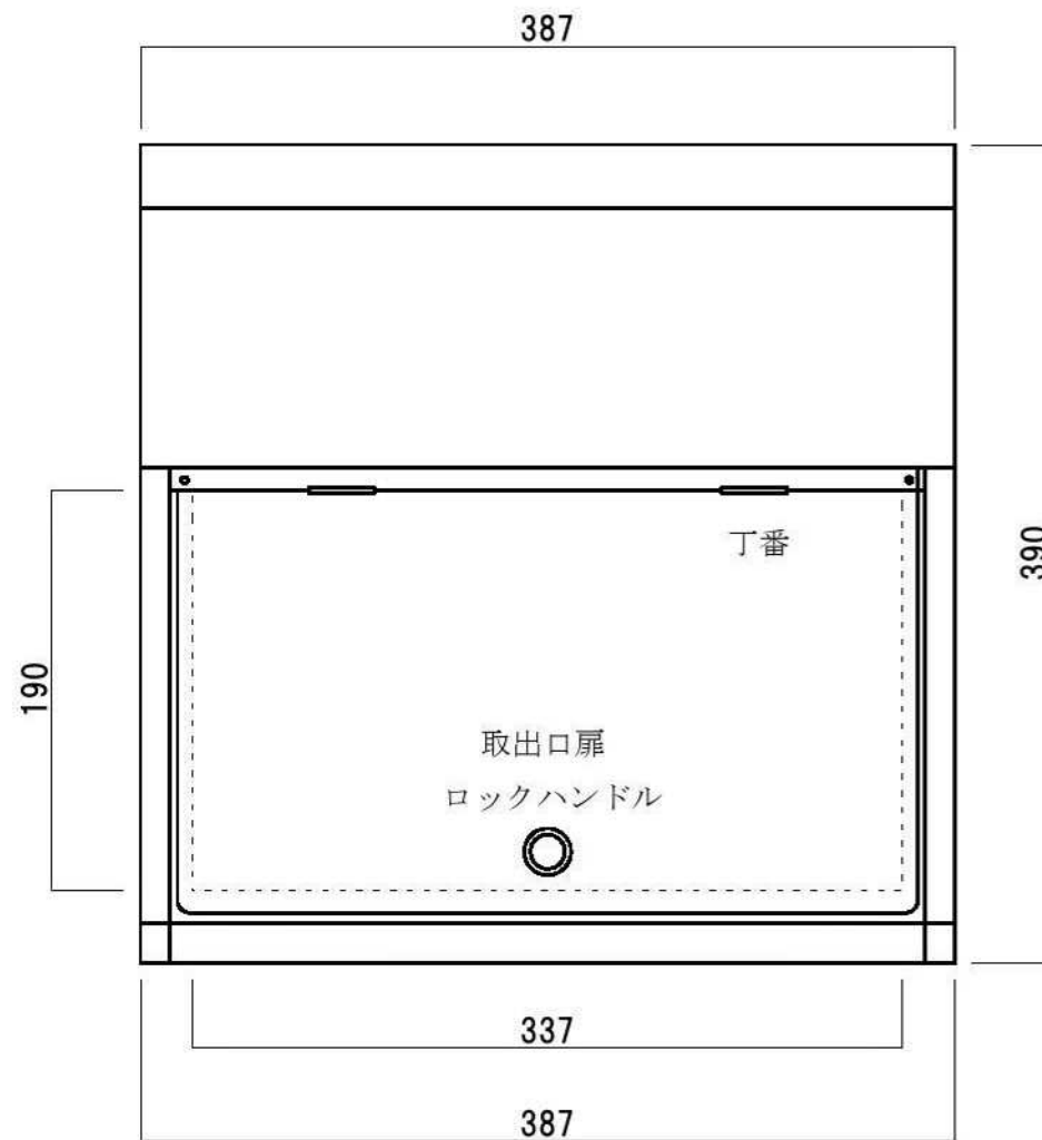
裏面図
