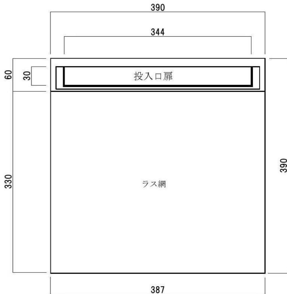
正面図
