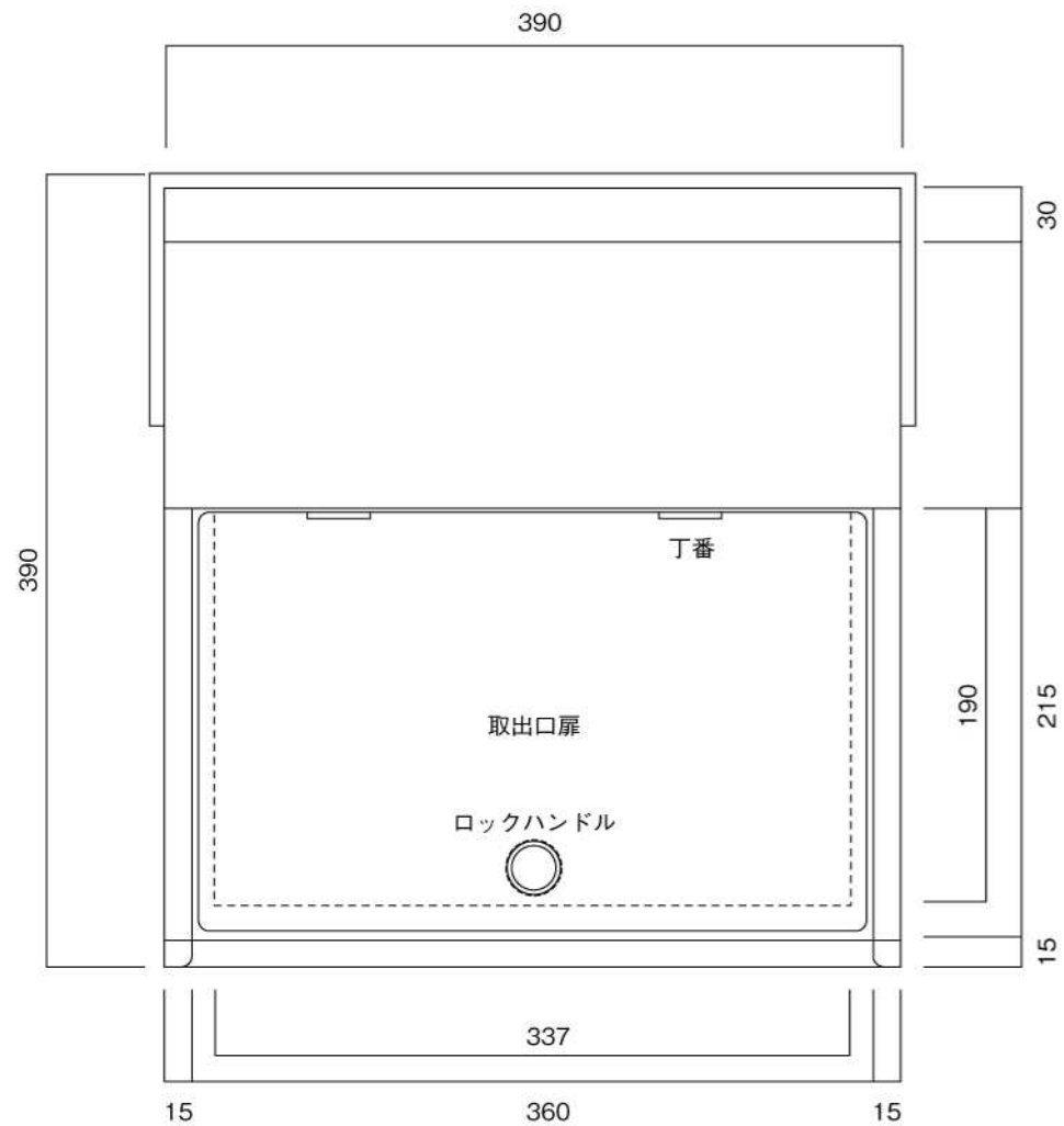
裏面図
