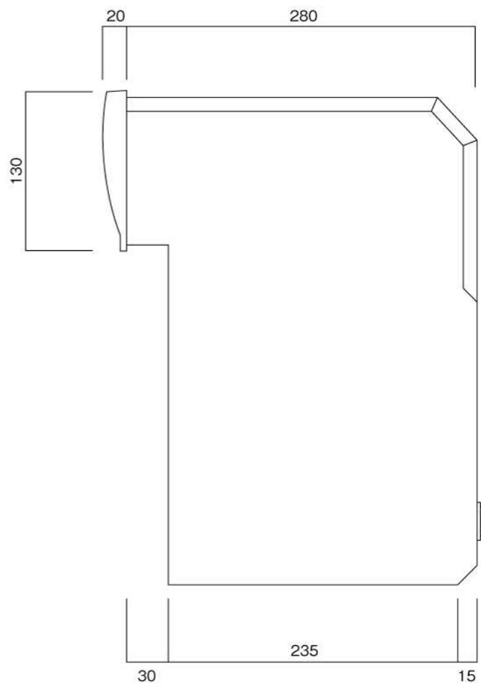
側面図
