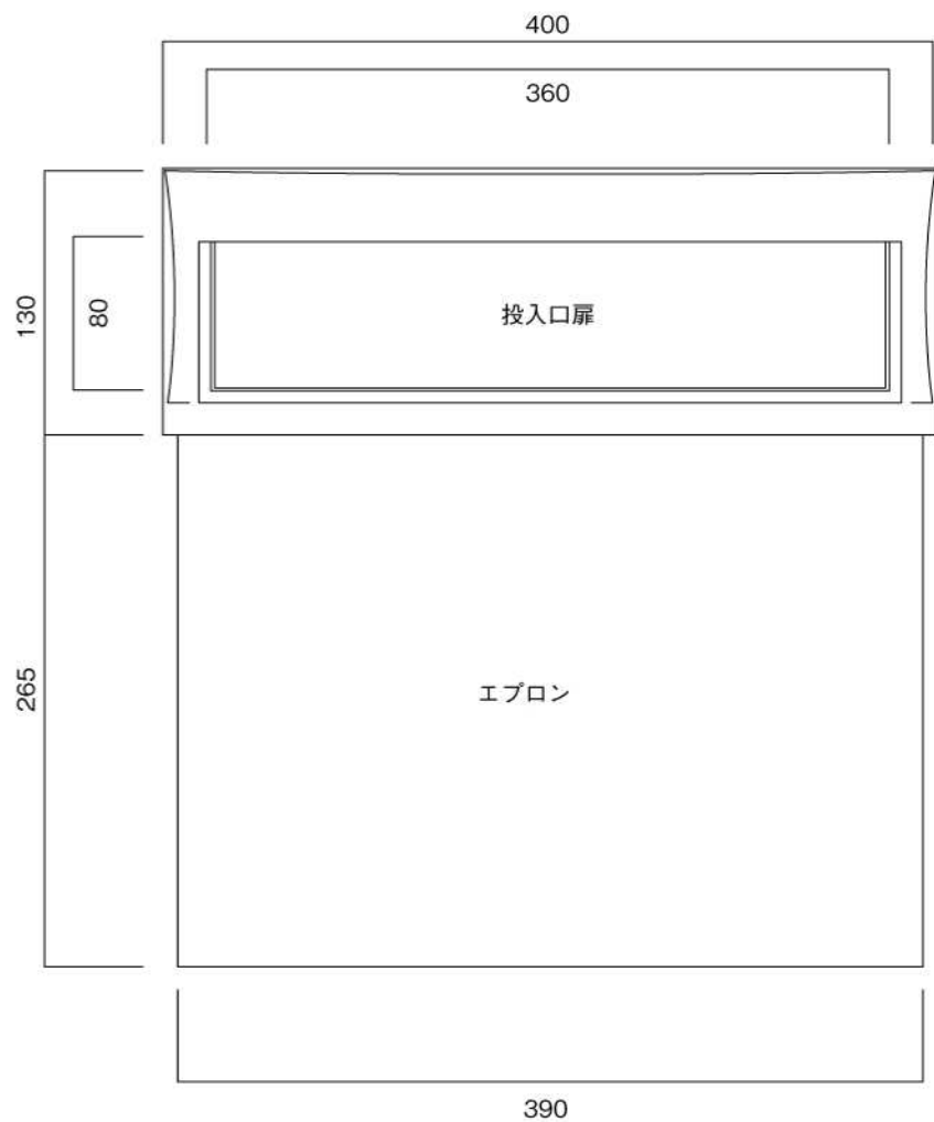
正面図
