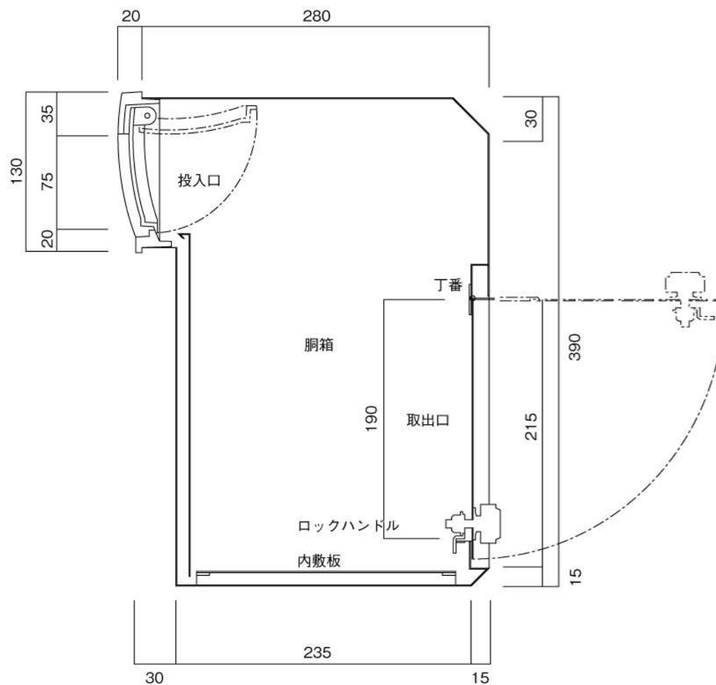
縦断面図
