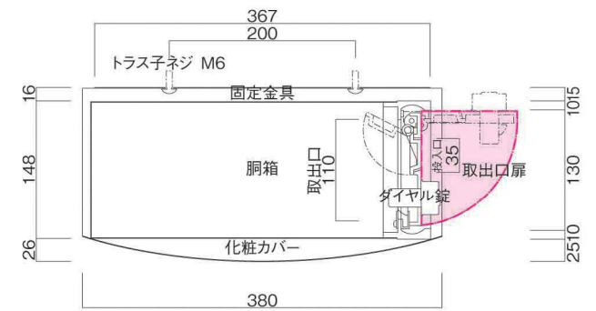
横断面図
