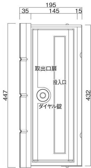
右側面図
