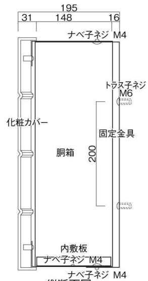
縦断面図
