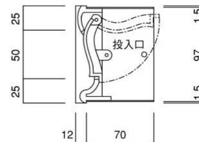
縦断面図
