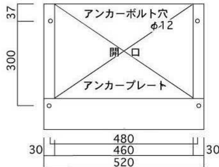
底面図
