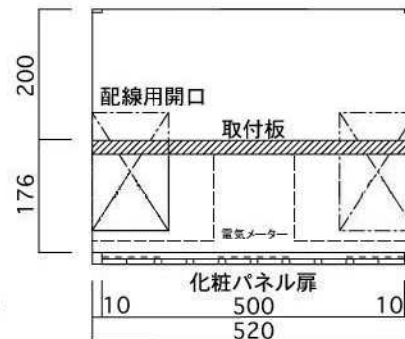
横断面図
