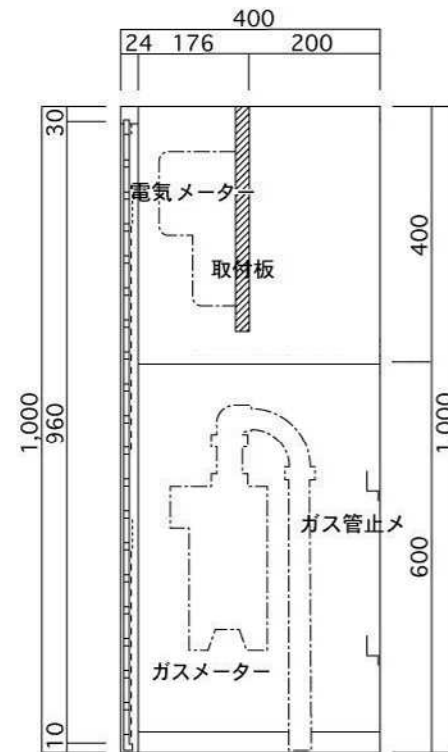
側面図
