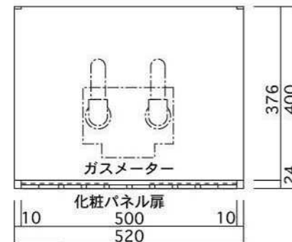
横断面図
