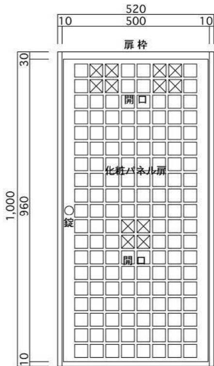
正面図
