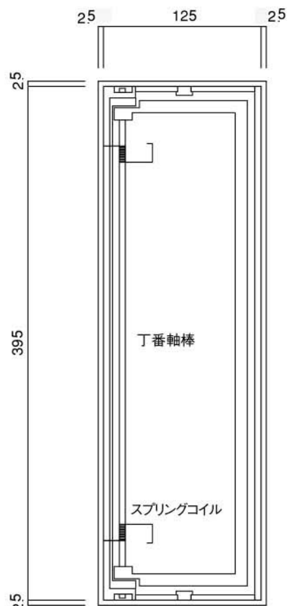
裏面図
