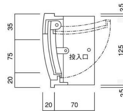
縦断面図
