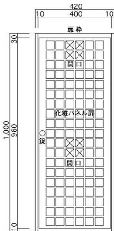
正面図
