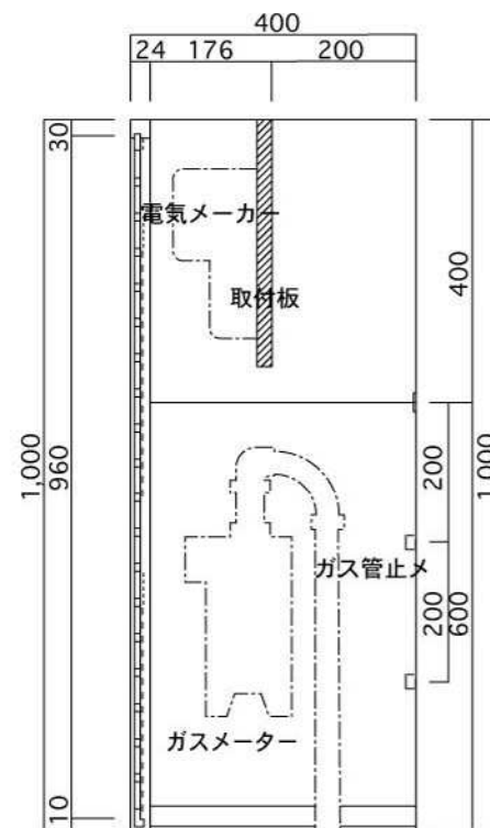
縦断面図
