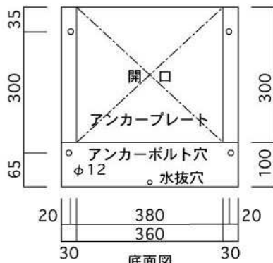
底面図
