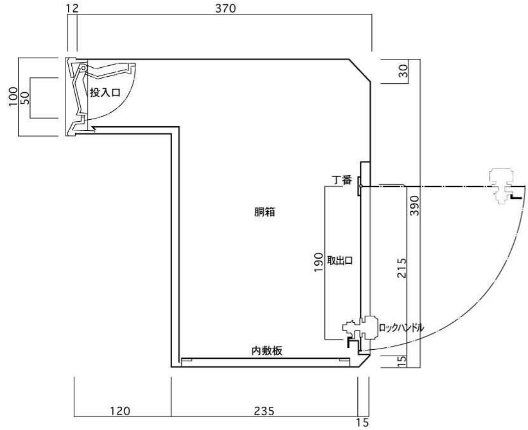
縦断面図
