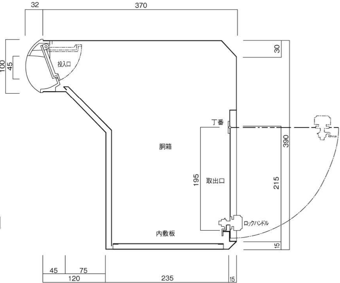
縦断面図
