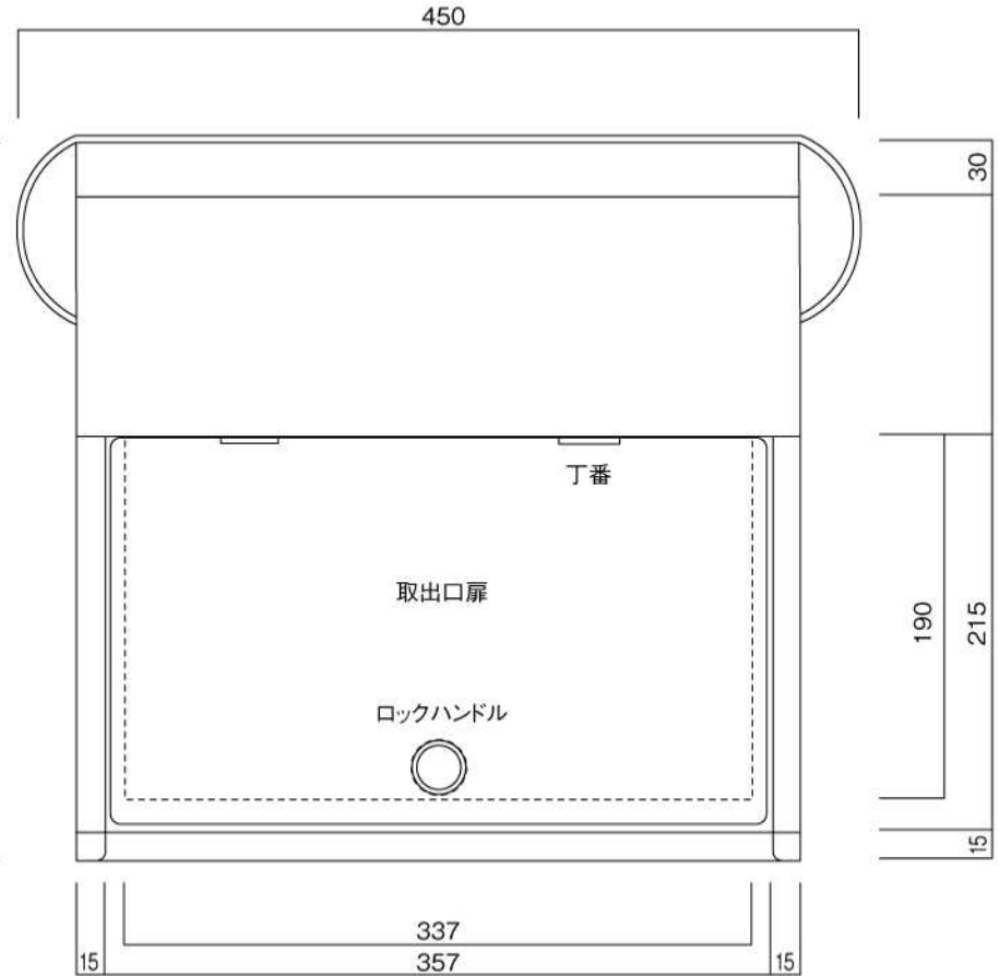
裏面図
