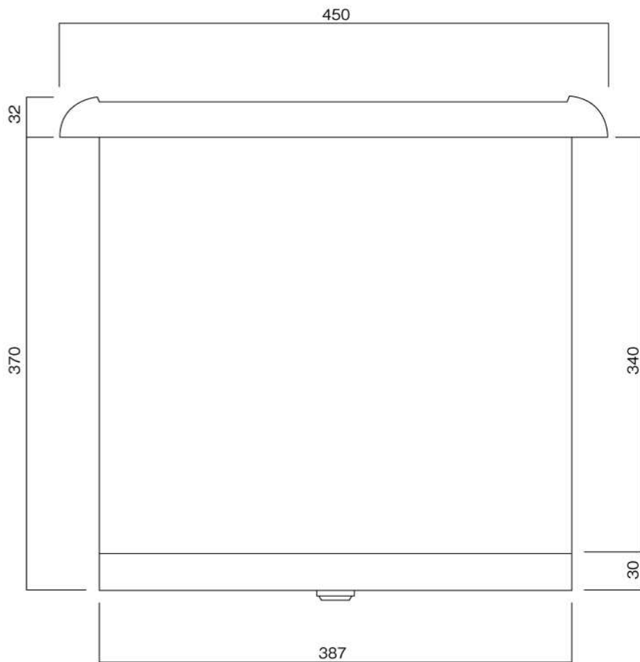
平面図
