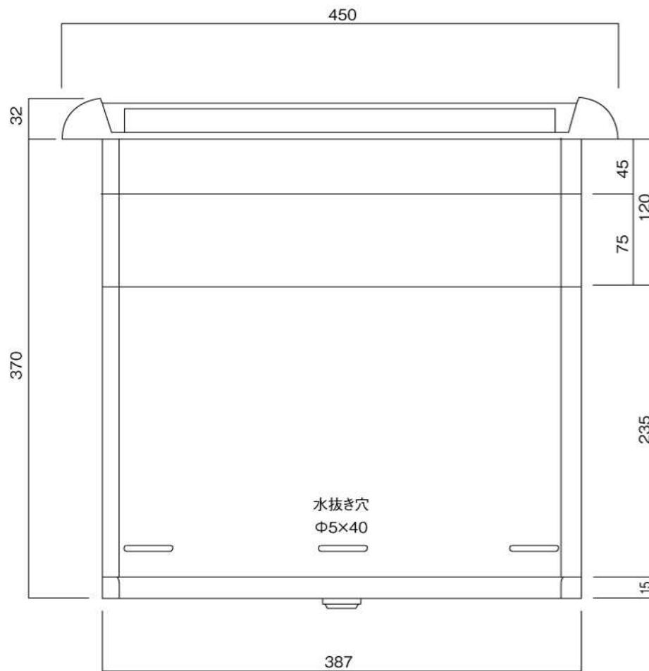
底面図
