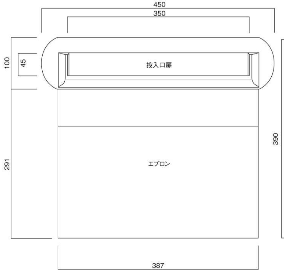
正面図
