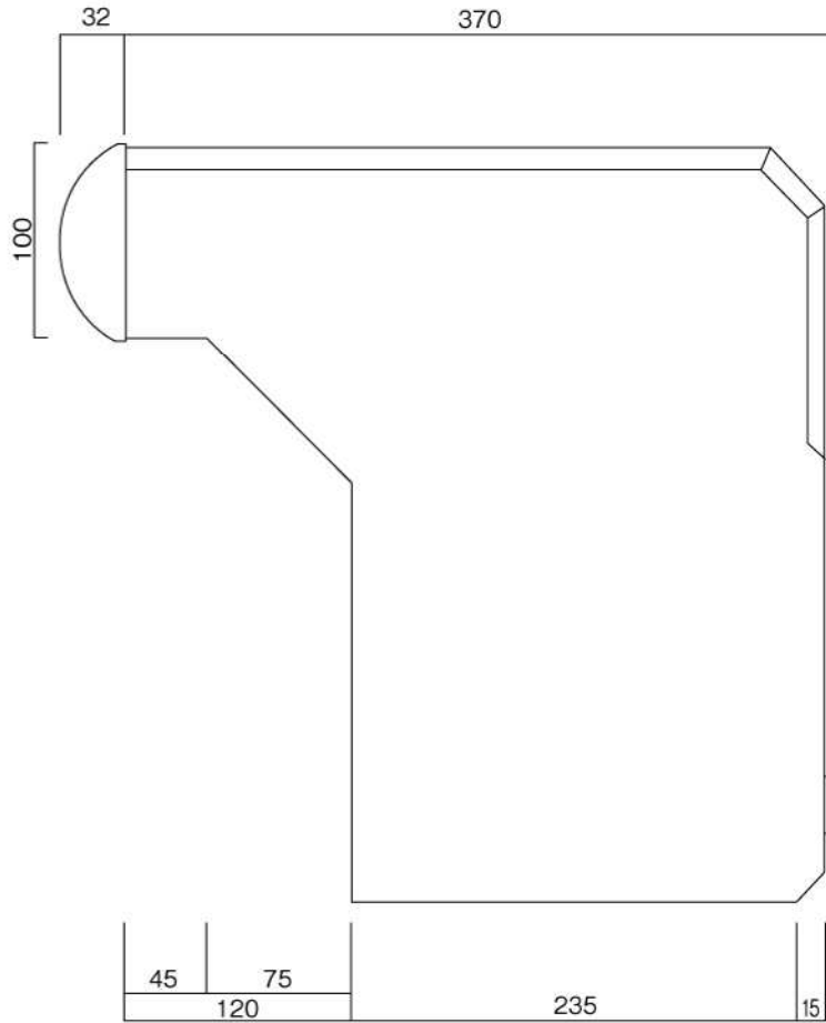
側面図
