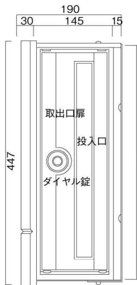
左側面図
