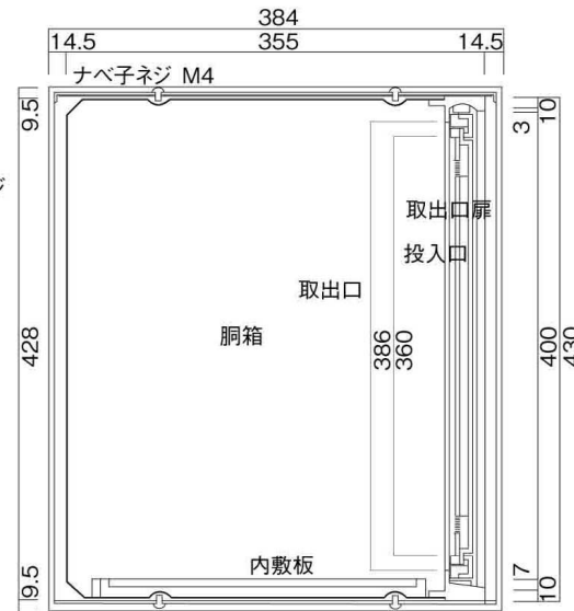
縦断面図
