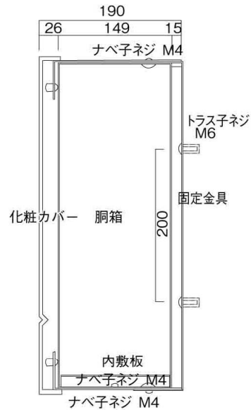
縦断面図
