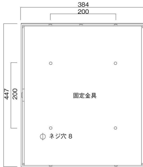
裏面図
