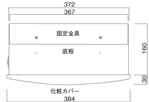
底面図
