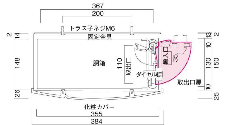
横断面図
