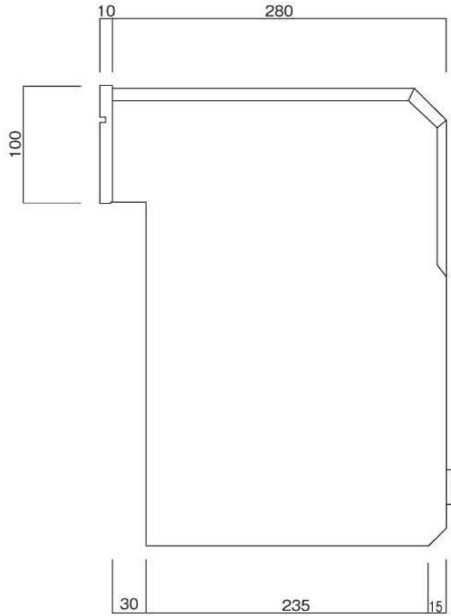
側面図
