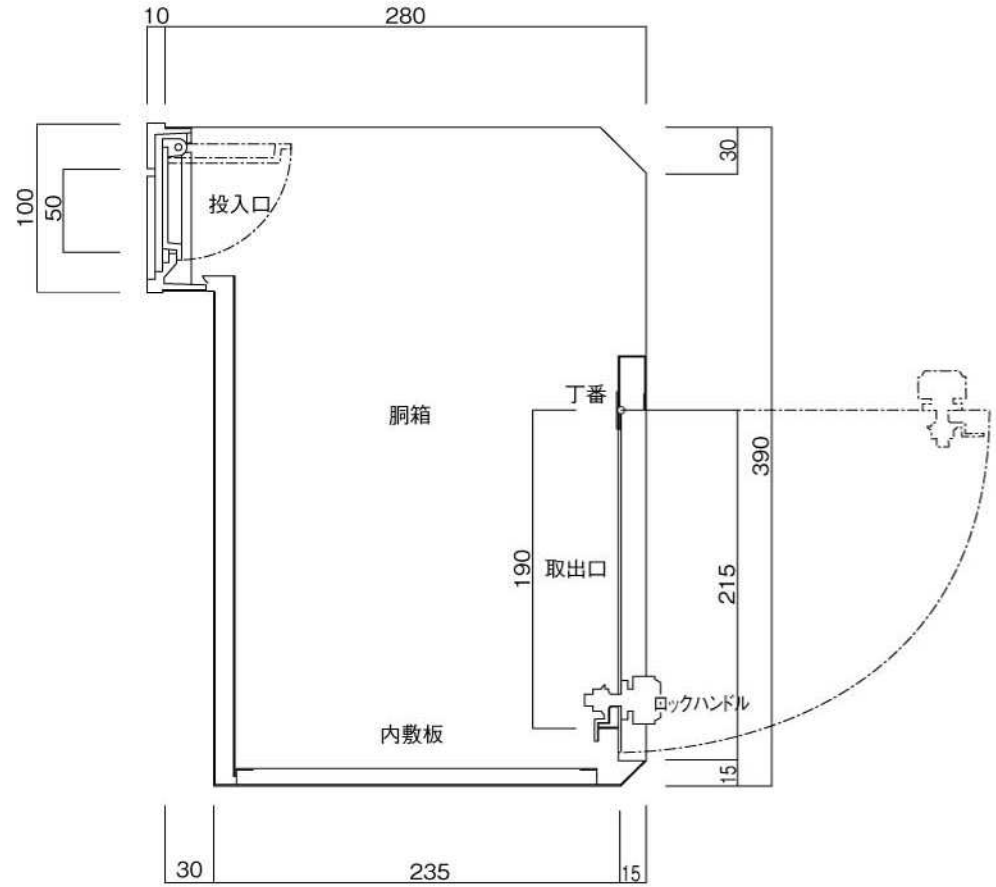
縦断面図
