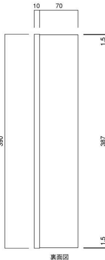
裏面図
