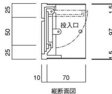
縦断面図
