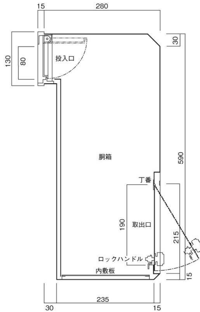
縦断面図
