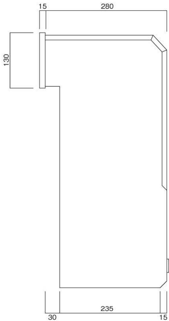
側面図
