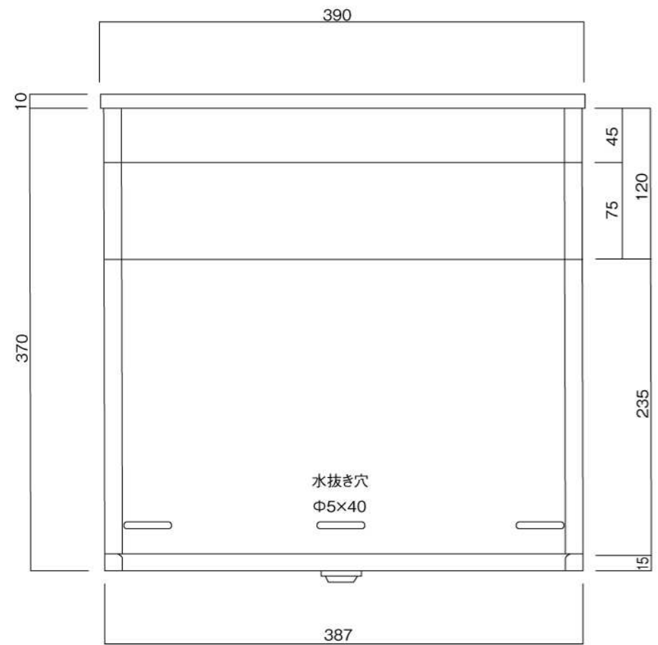
底面図
