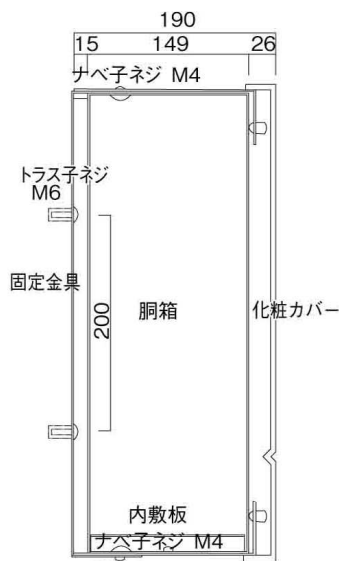
縦断面図
