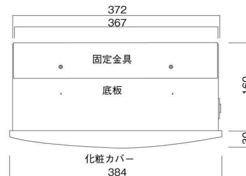
底面図
