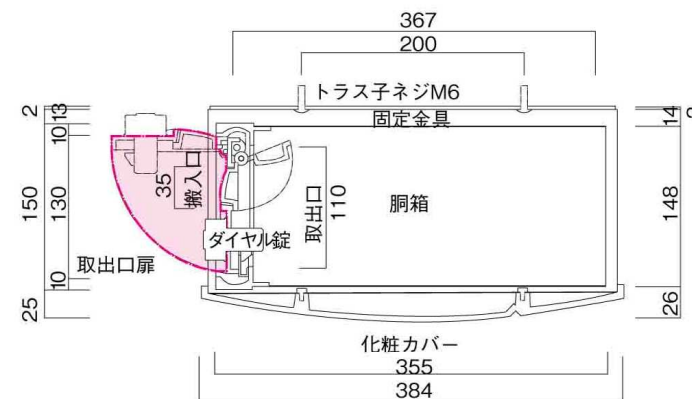
横断面図
