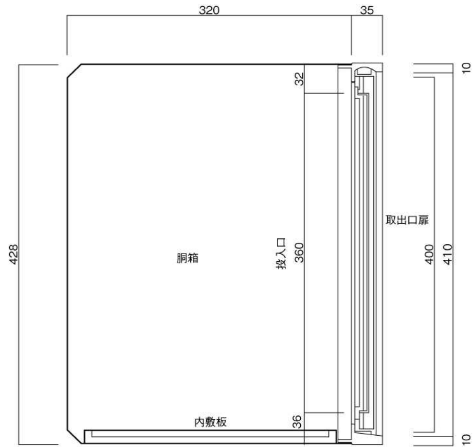
縦断面図
