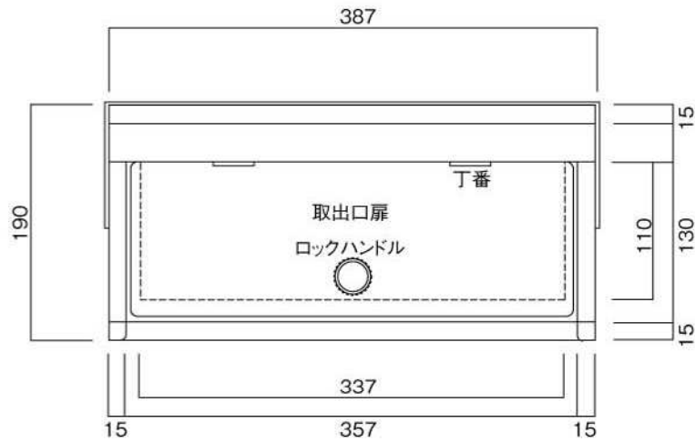
裏面図
