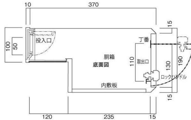
縦断面図
