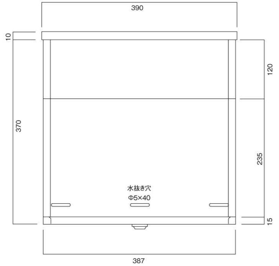
底面図
