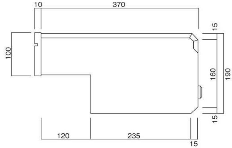
側面図
