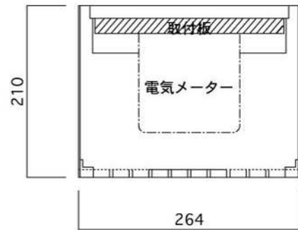
横断面図
