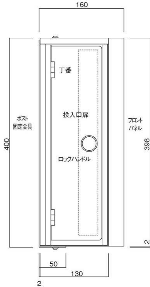
左側面図
