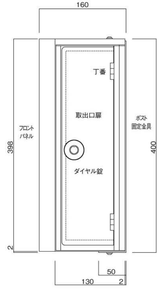
右側面図
