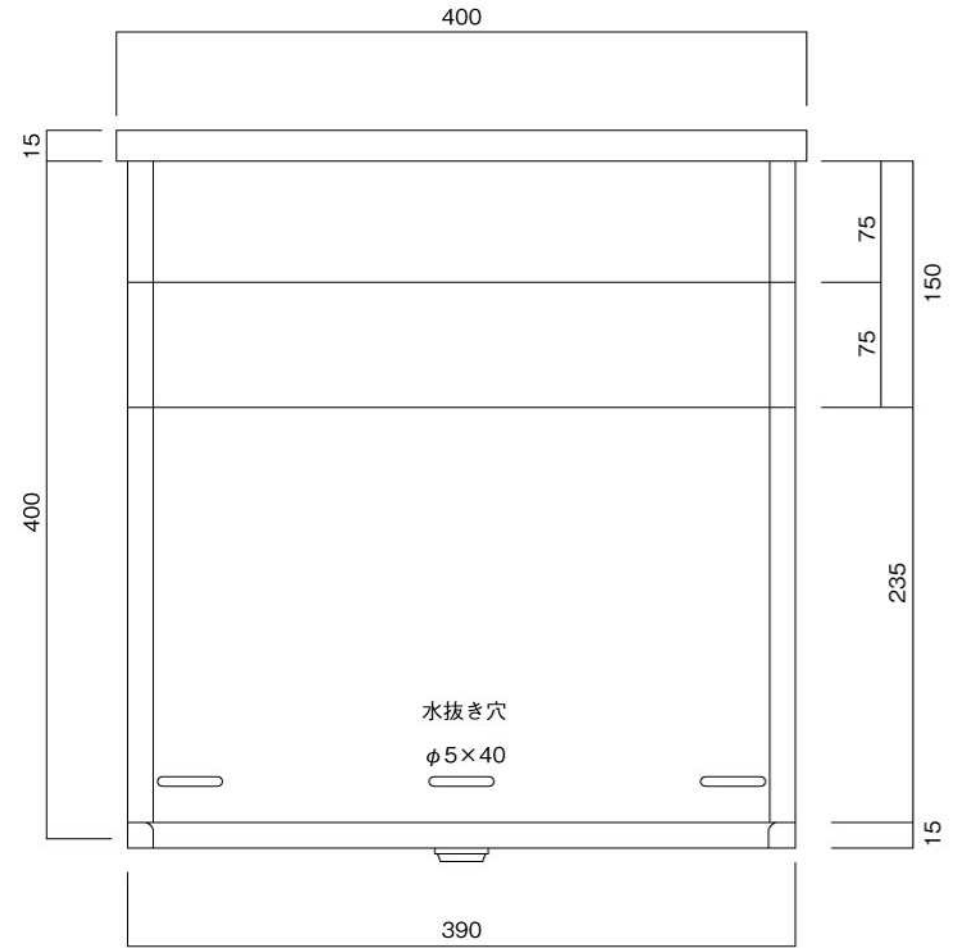
底面図
