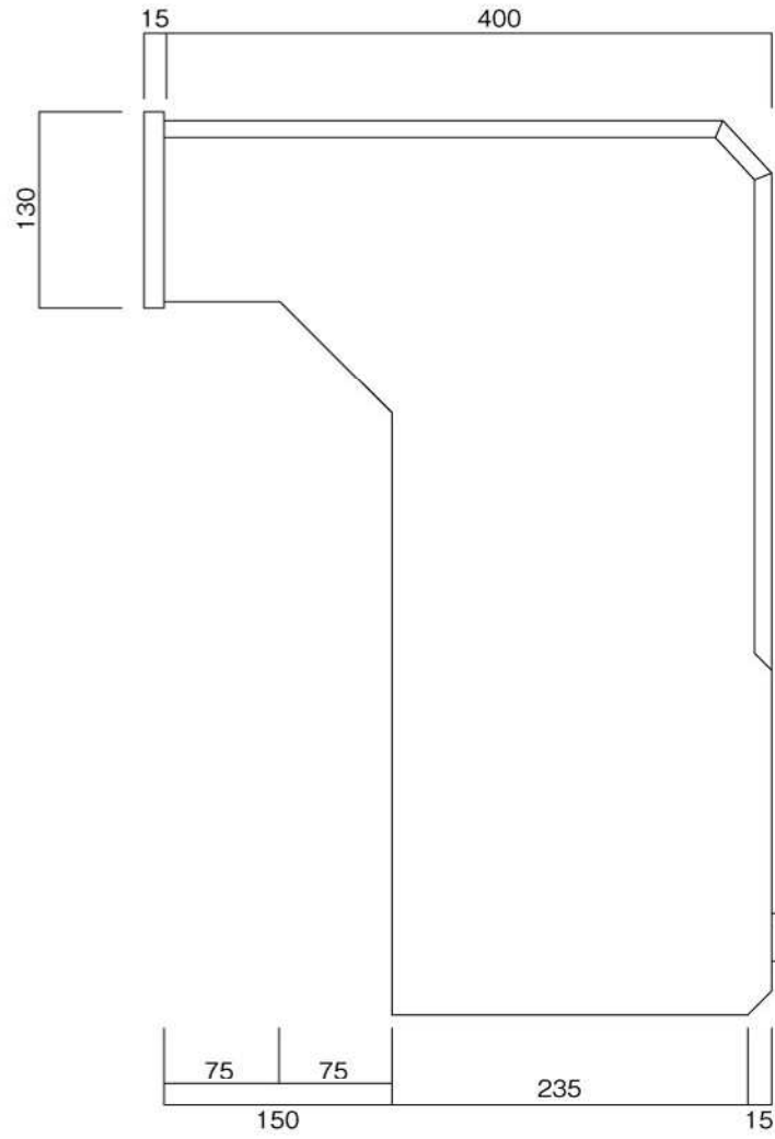
側面図
