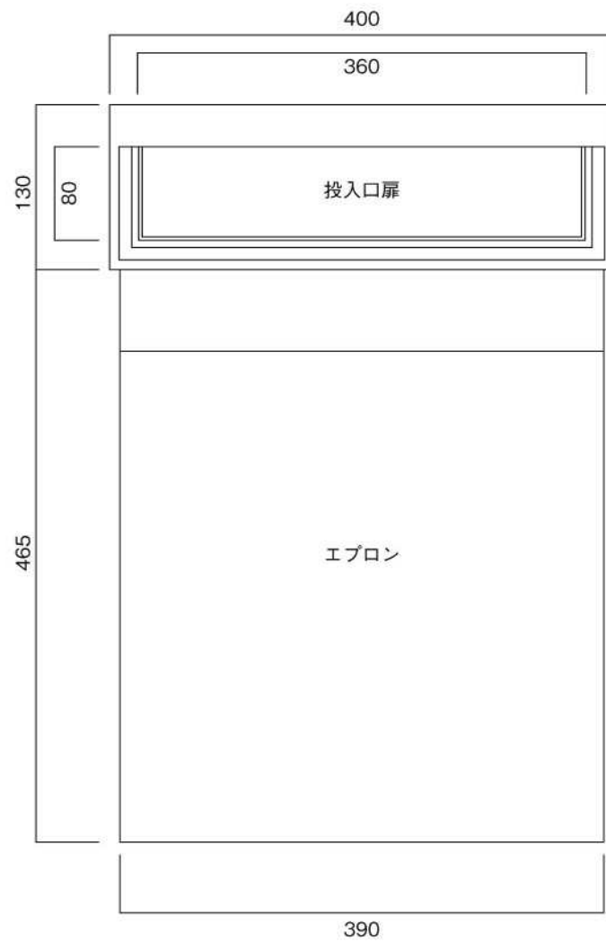
正面図
