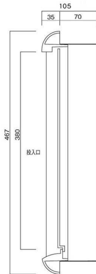
縦断面図
