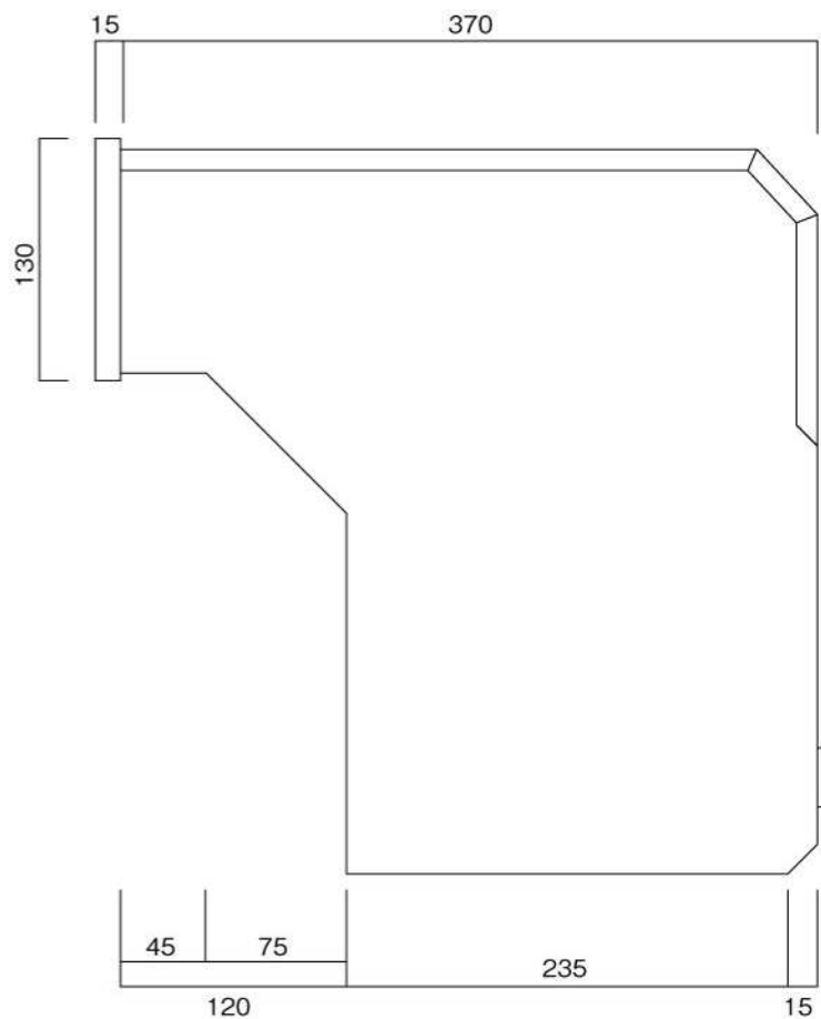
側面図
