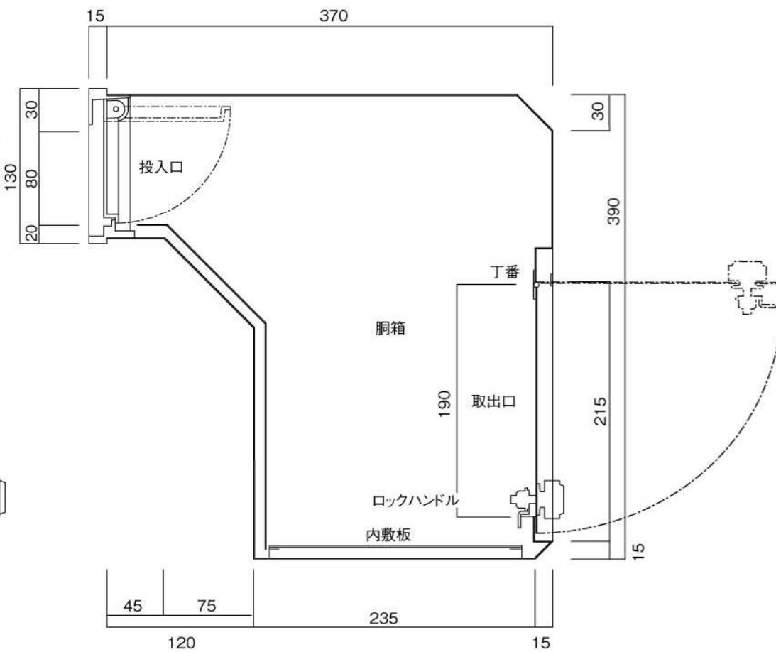
縦断面図
