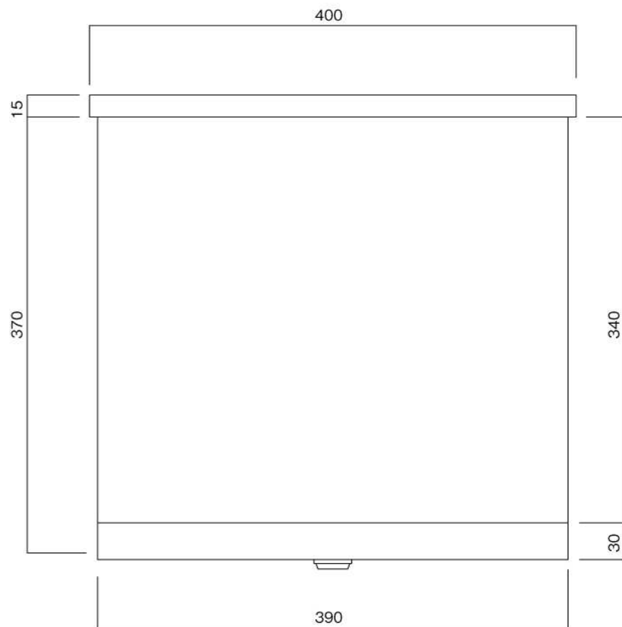
平面図
