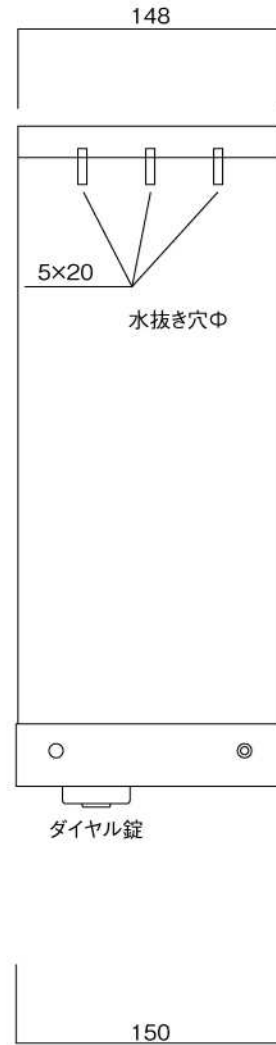
底面図
