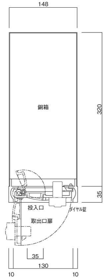
横断面図
