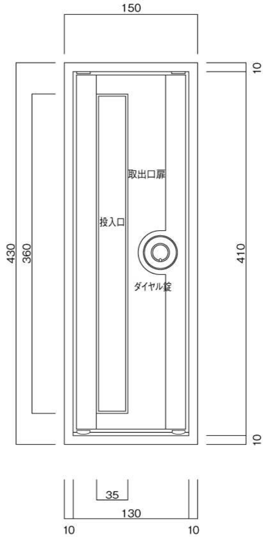
正面図
