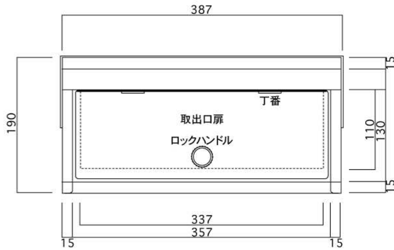
裏面図
