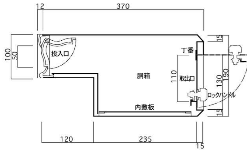
縦断面図
