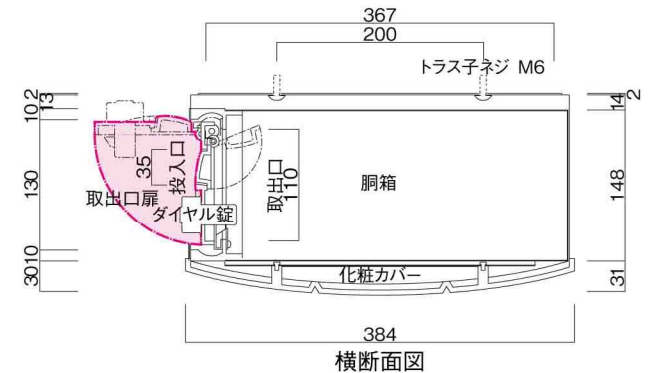
横断面図
