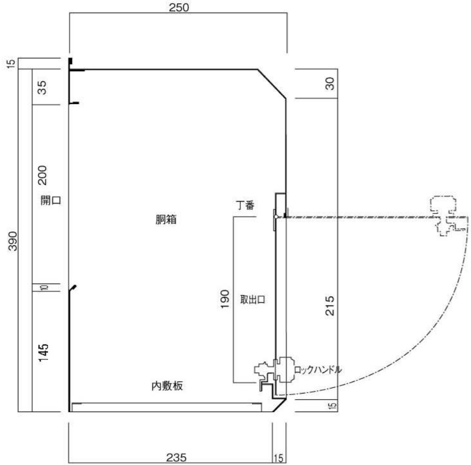
縦断面図
