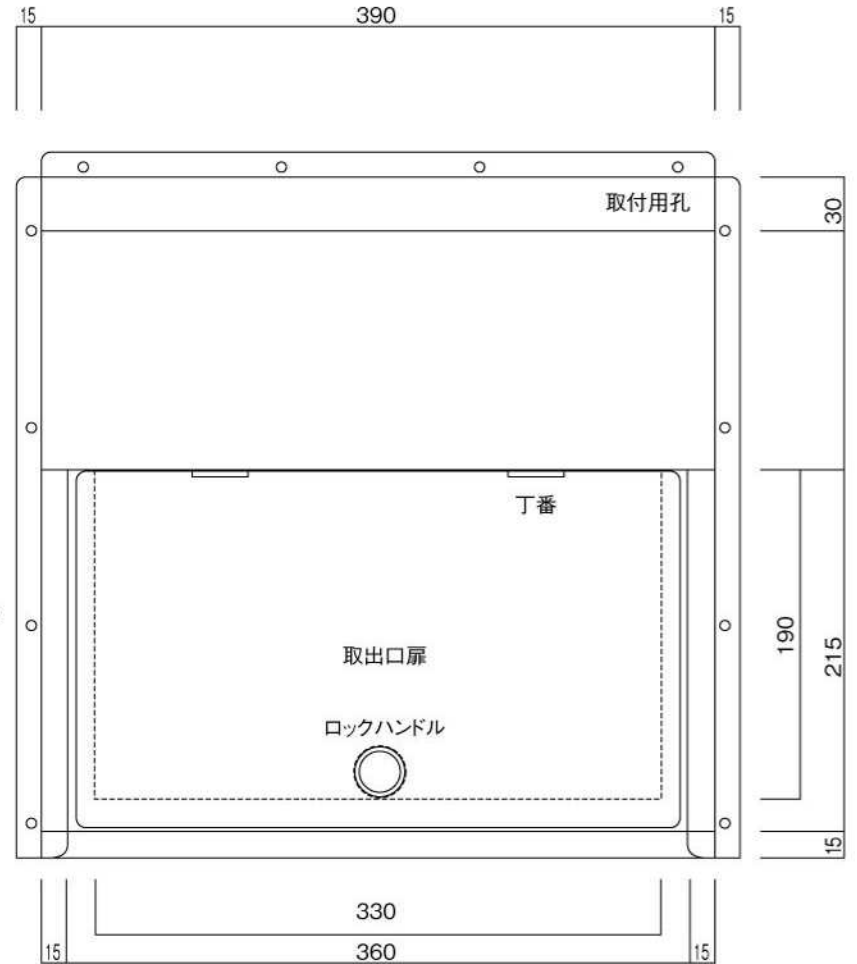
裏面図
