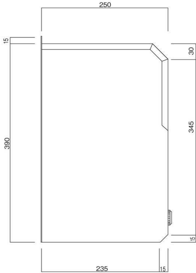
側面図
