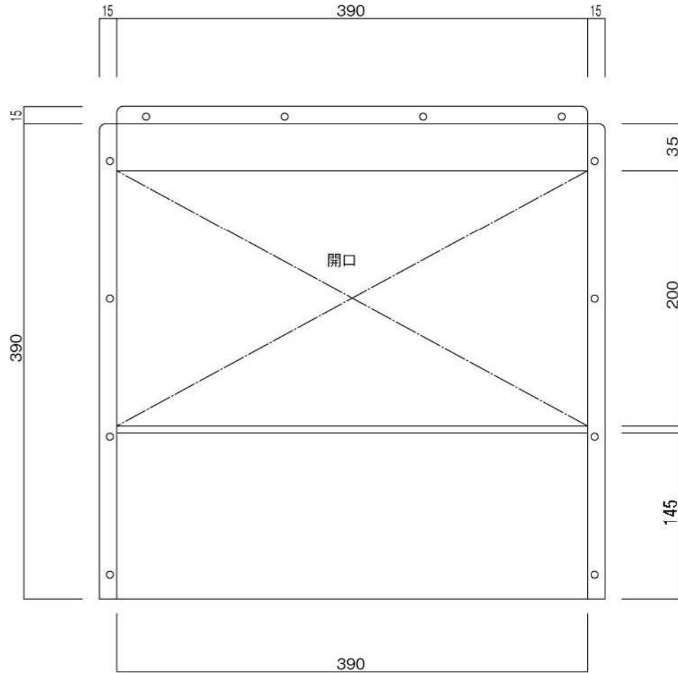
正面図
