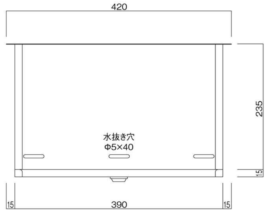
底面図
