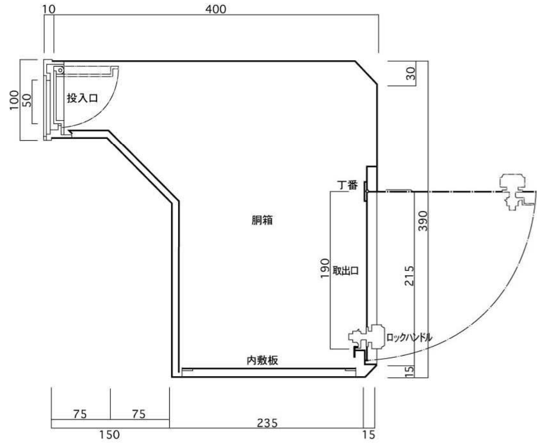
縦断面図
