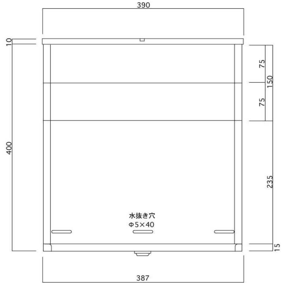
底面図
