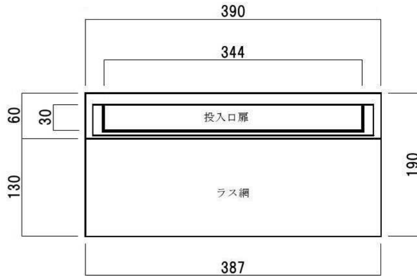
正面図
