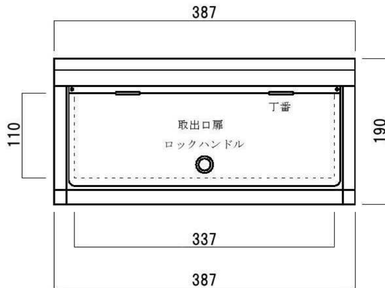
裏面図
