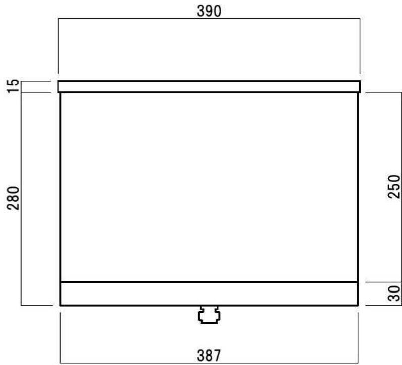
平面図
