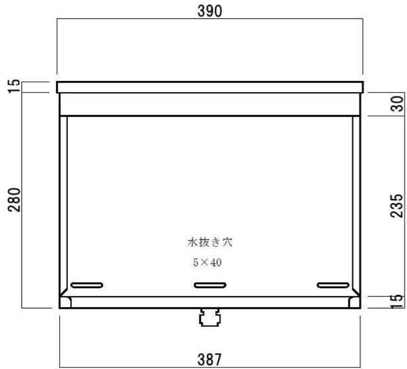
底面図
