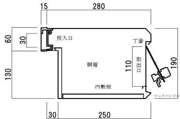
縦断面図
