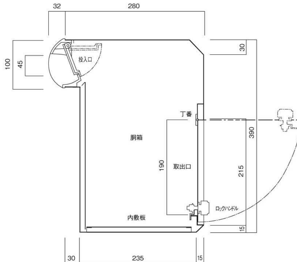
縦断面図
