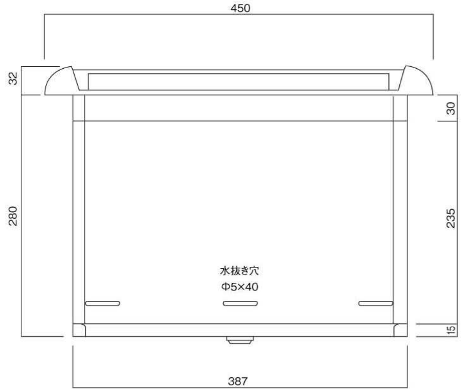
底面図
