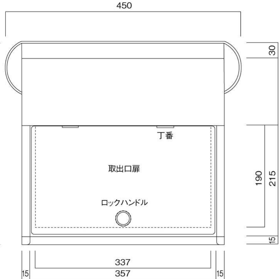
裏面図
