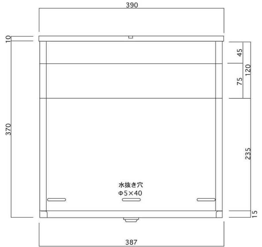
底面図
