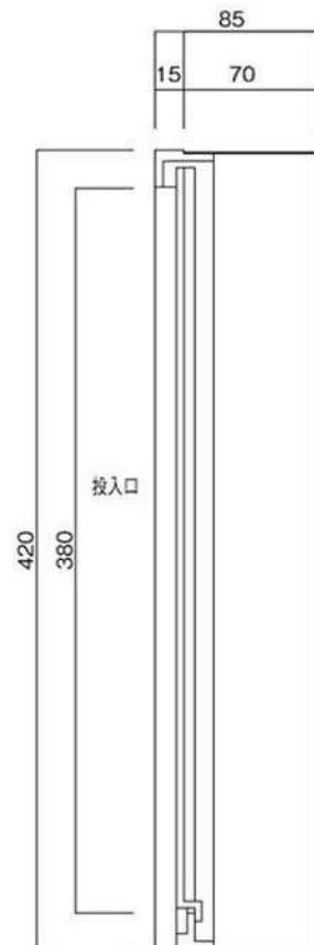
縦断面図
