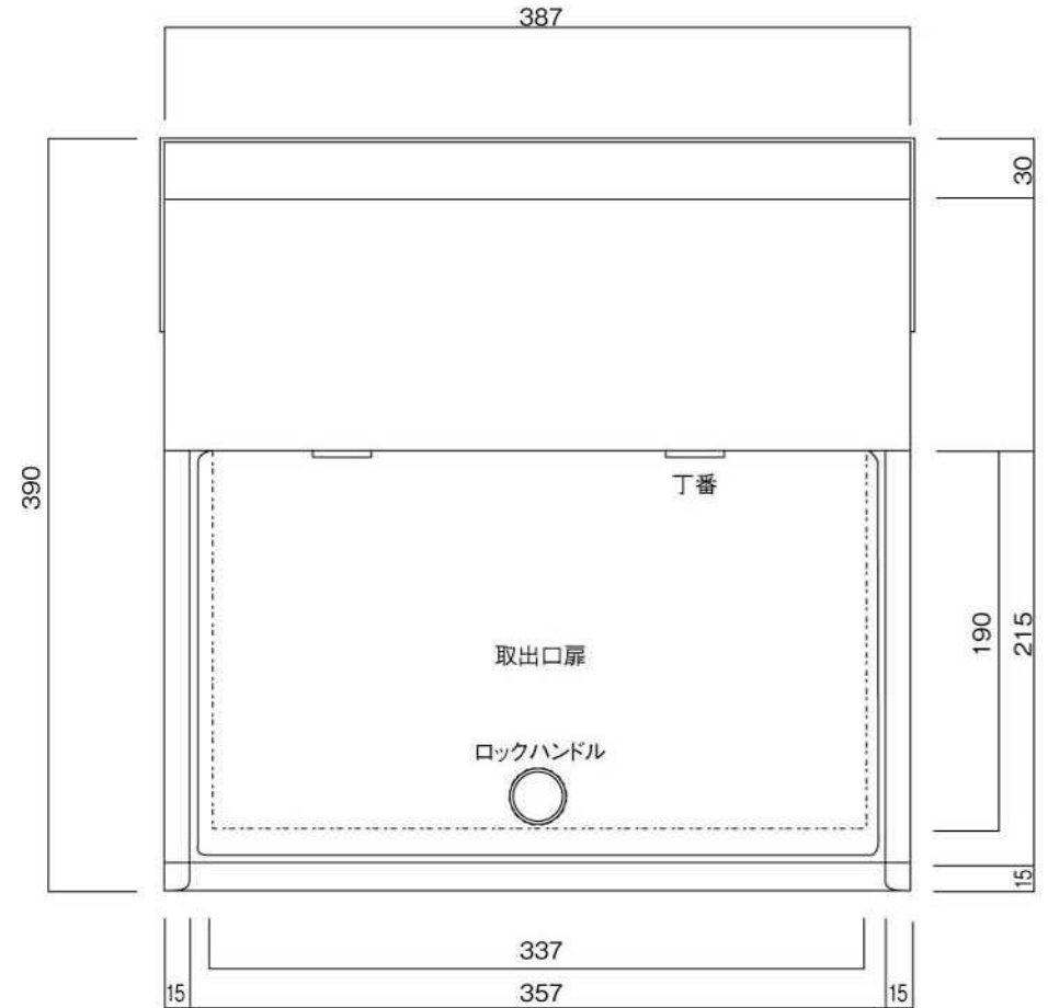
裏面図
