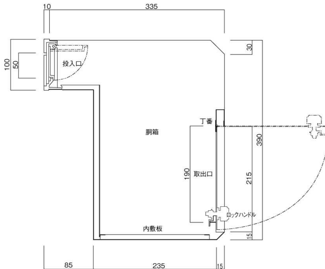
縦断面図
