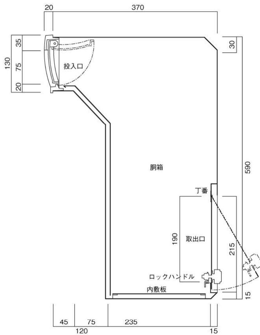
縦断面図
