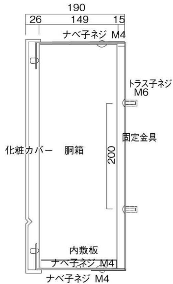
縦断面図
