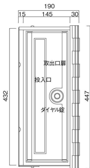
左側面図
