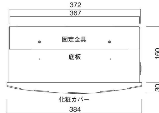
底面図
